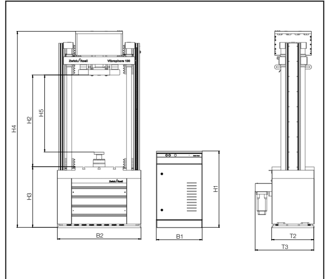
Zeichnung: Vibrophore 100
